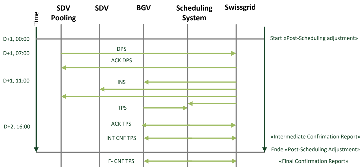
Abbildung 8: Fahrplanabstimmungsprozess
